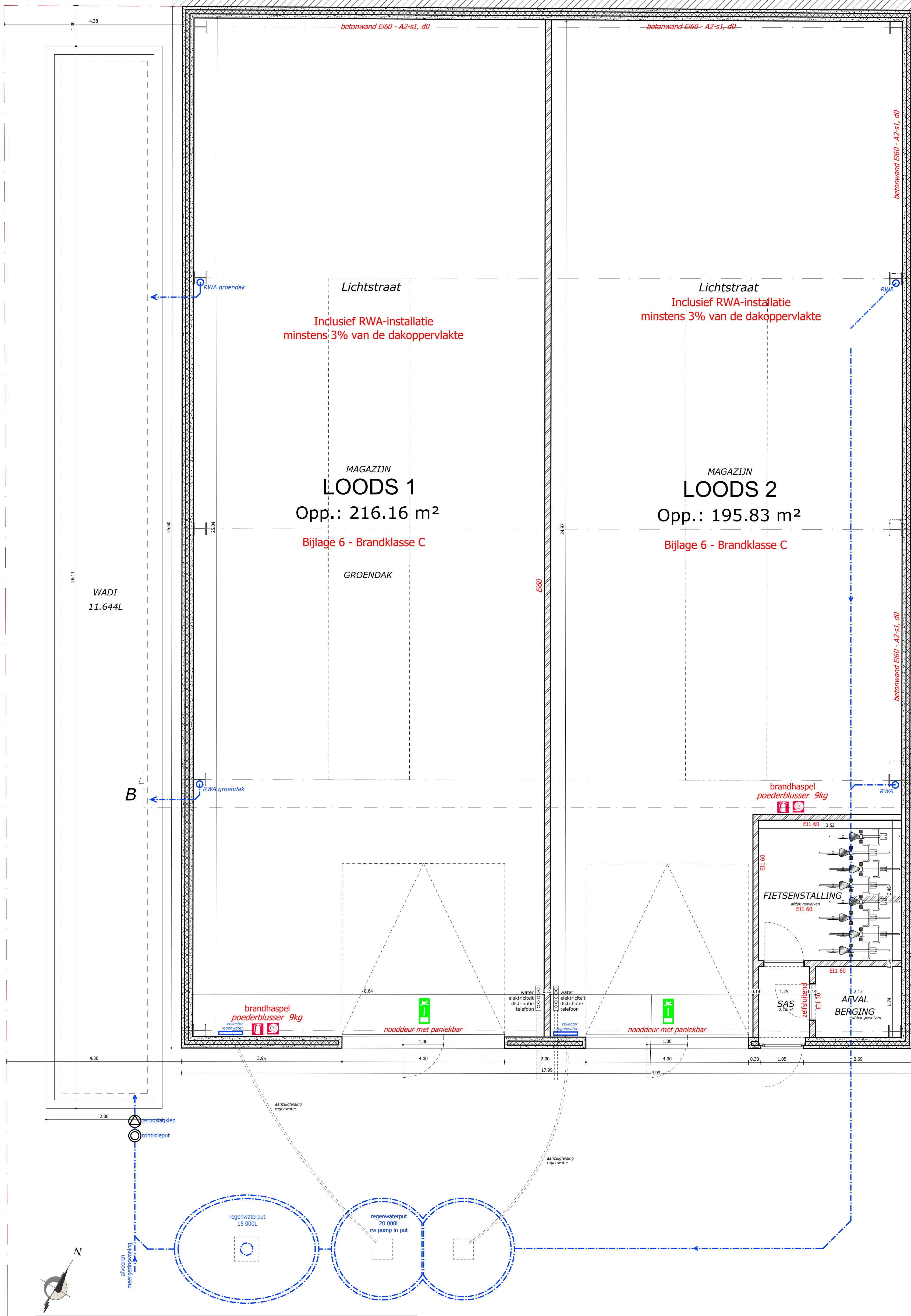
GELIJKVLOERS LOODS SCHAAL 1:50
